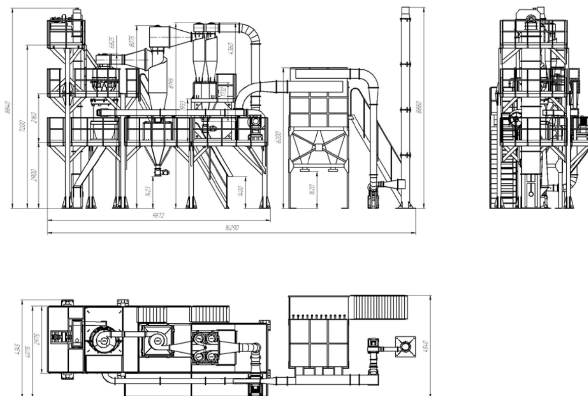
Рис. Один из вариантов компоновки (металлоконструкций) линии на базе мельницы Титан-М
