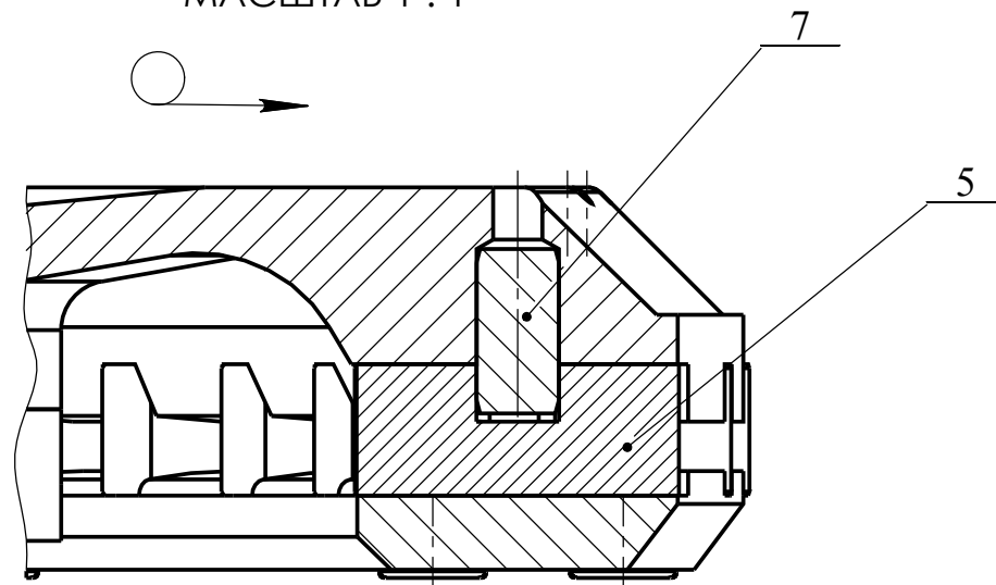
СЕЧЕНИЕ С-С МАСШТАБ 1 : 1
